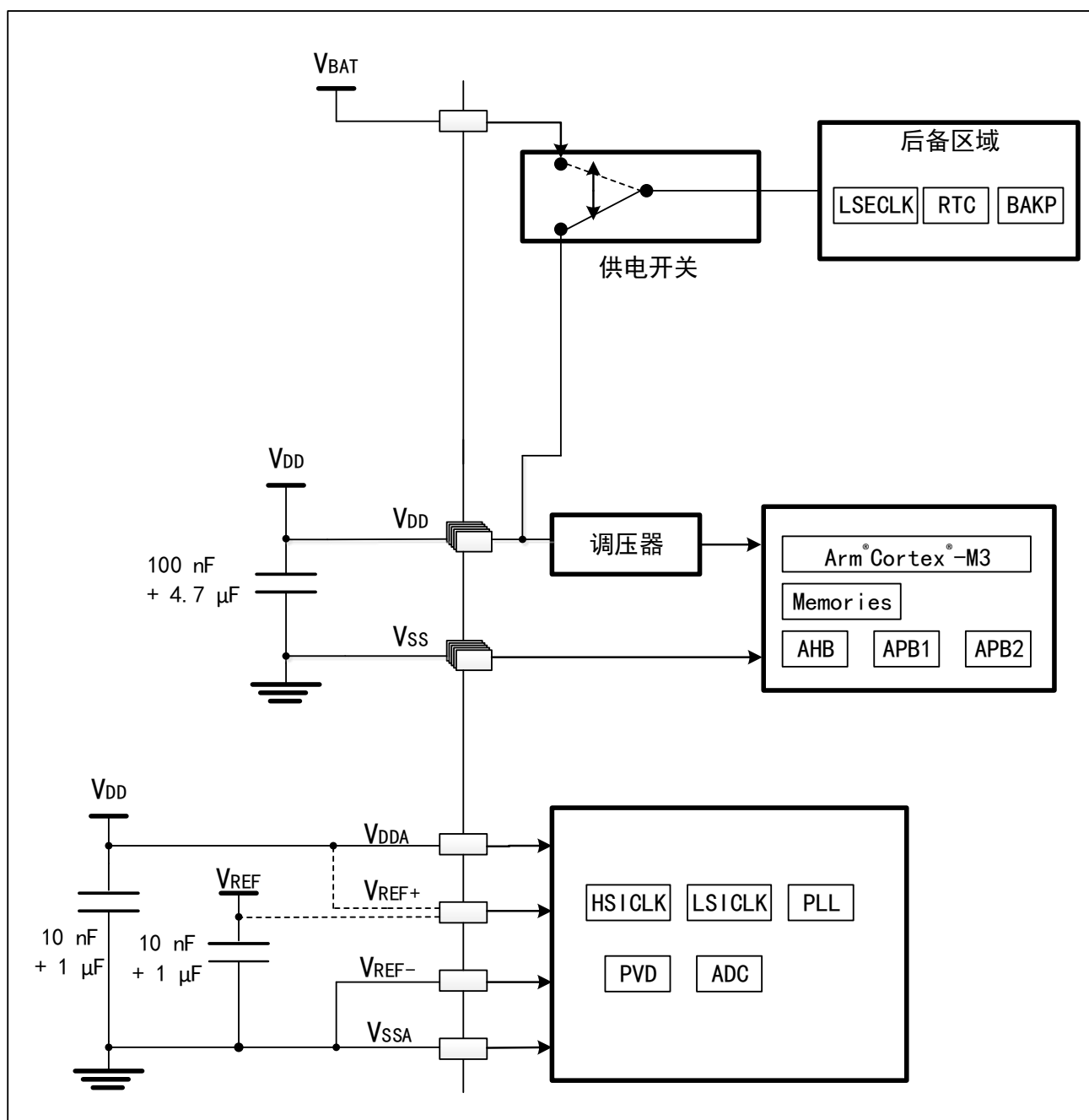
图8 供电方案
