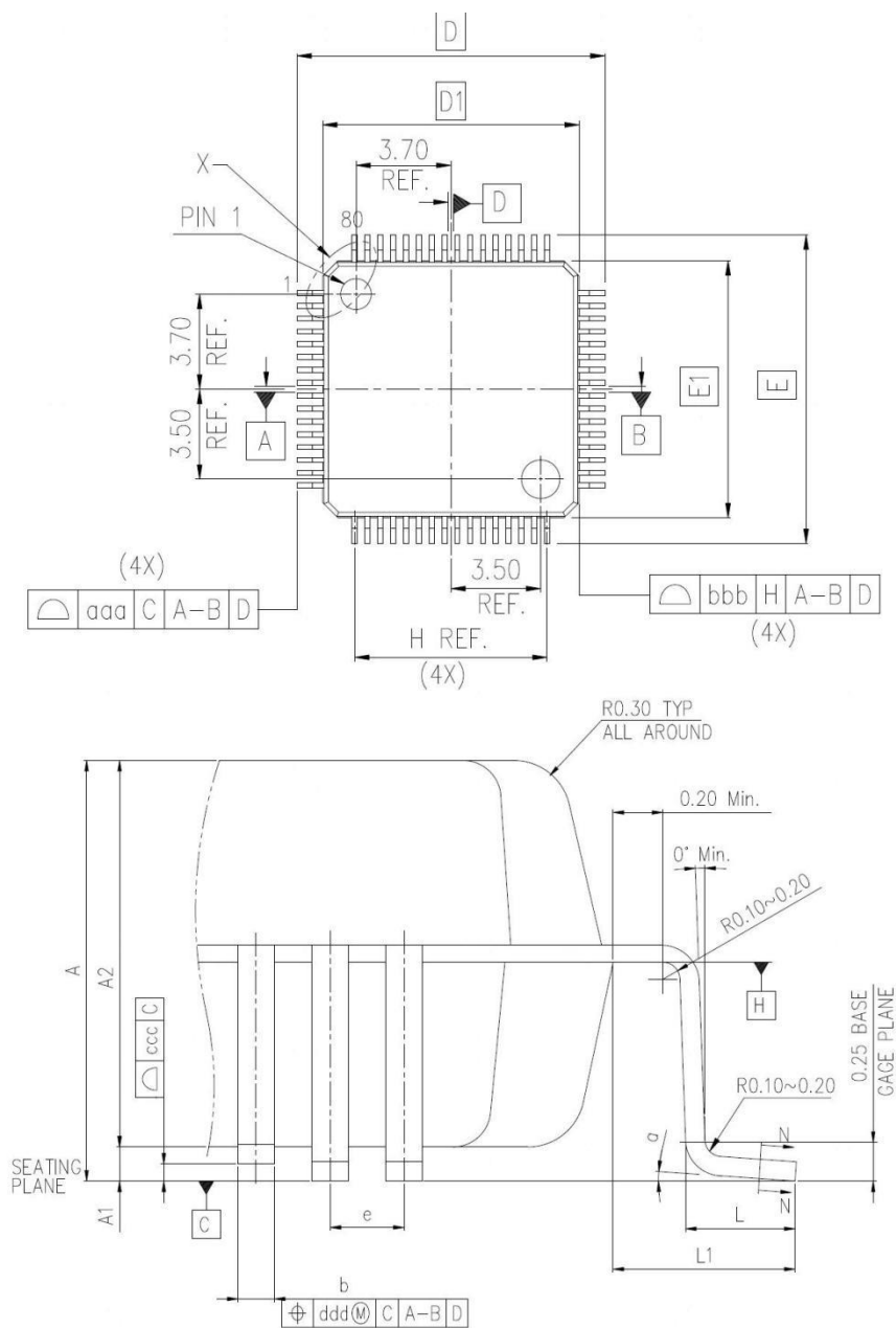
图25 LQFP64 封装图
