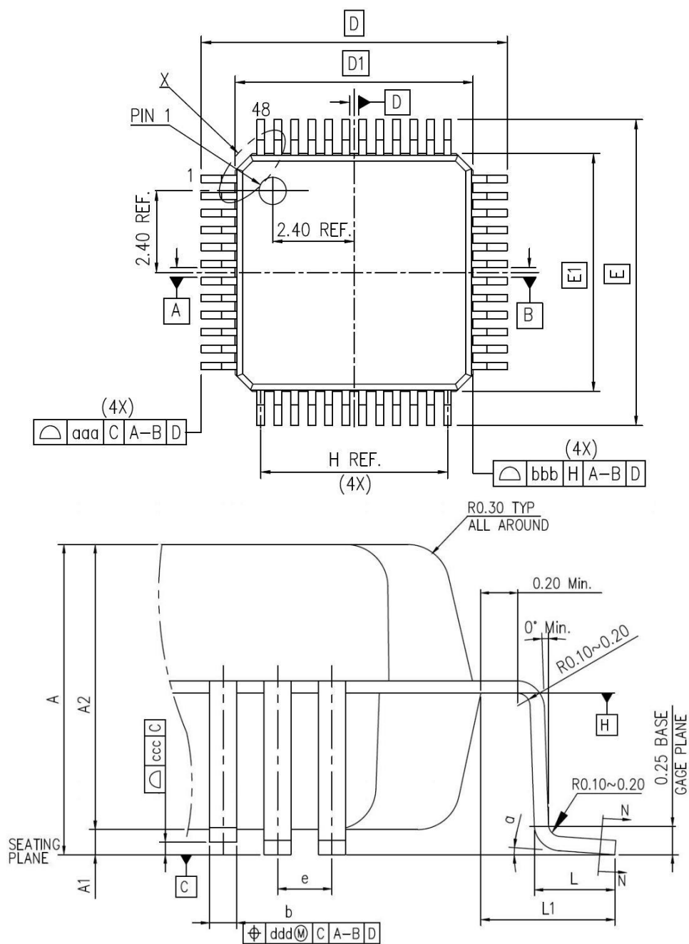
图28 LQFP48 封装图
