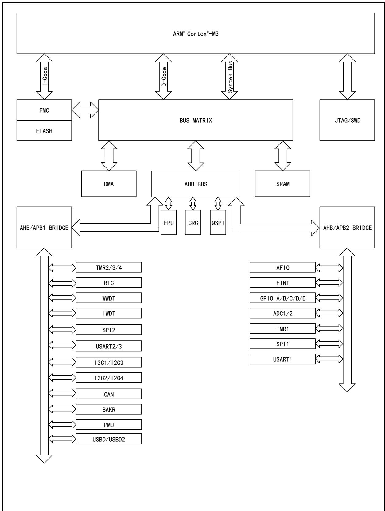
图5 APM32F103x4x6x8xB 系列系统框图
