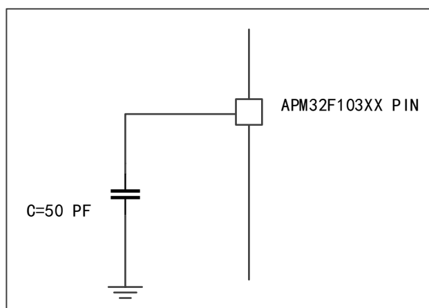
图9 测量引脚参数时的负载条件
