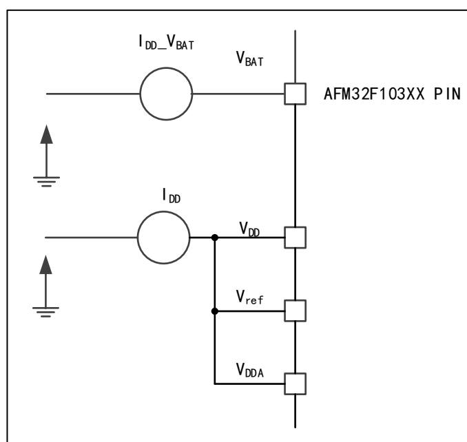
图11 电流消耗测量方案
