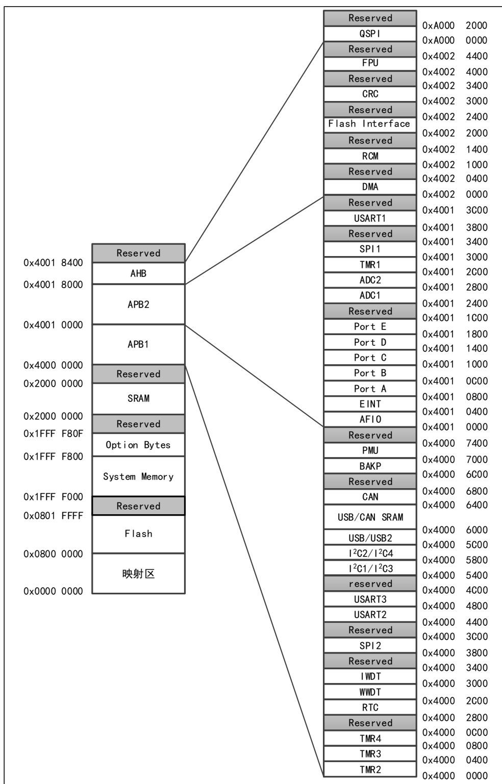
图7 APM32F103x4x6x8xB 系列地址映射图
