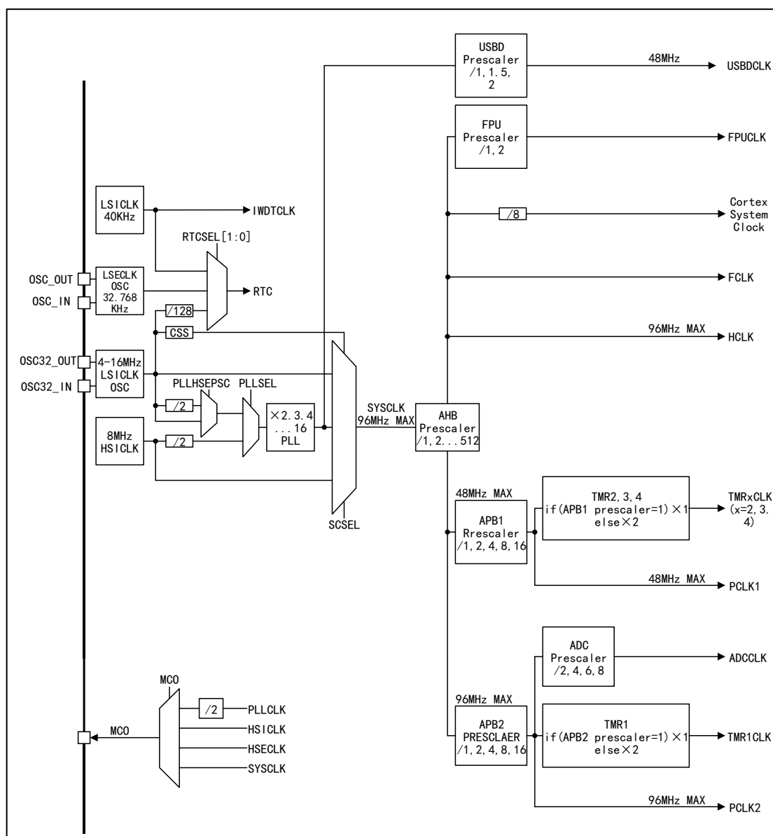
图6 APM32F103x4x6x8xB 系列时钟树
