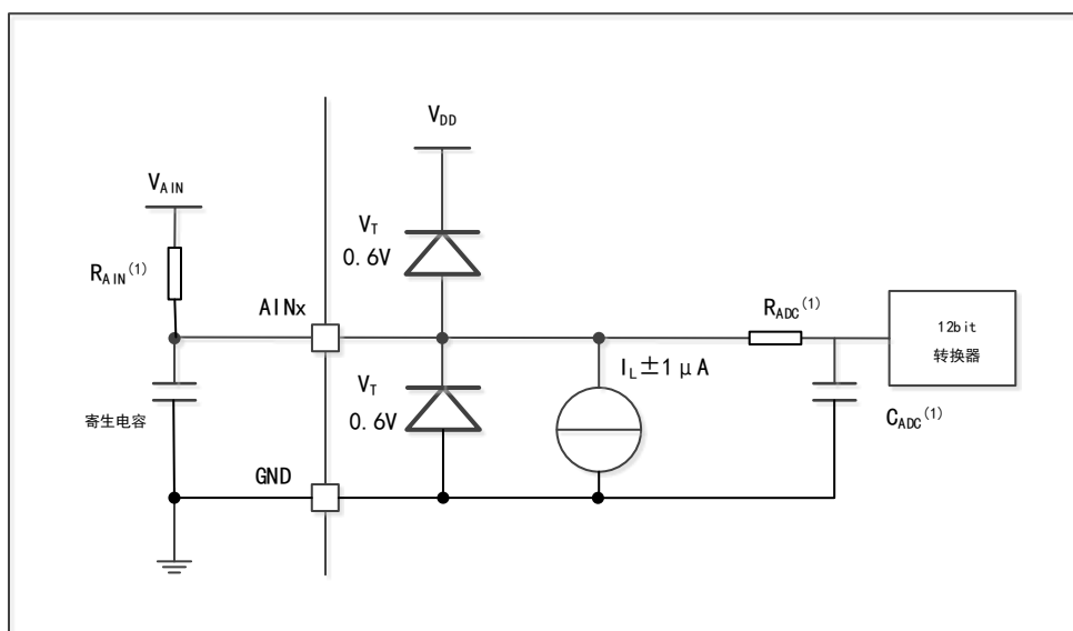
图20 ADC 的典型应用
