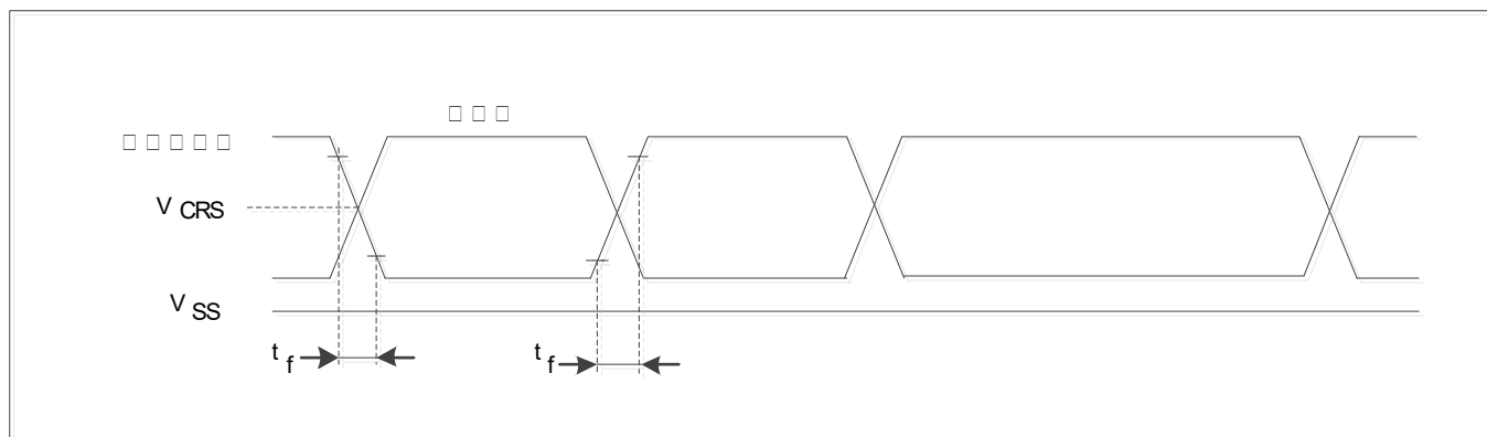
图19 USB D 时序：数据信号上升和下降的时间定义
