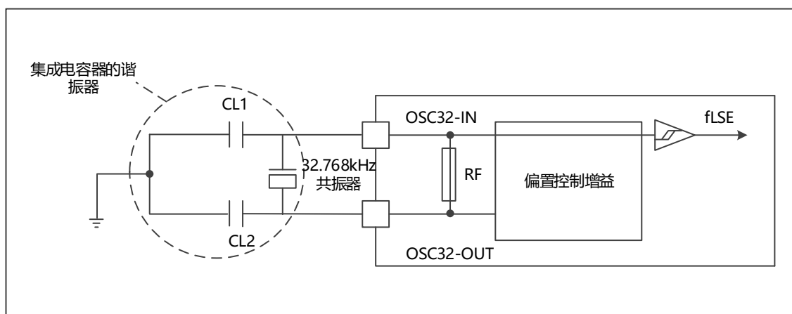
图13 使用 32.768kHz 的典型应用
